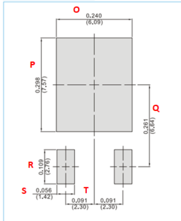
TO-252 Unit : inch(mm)
