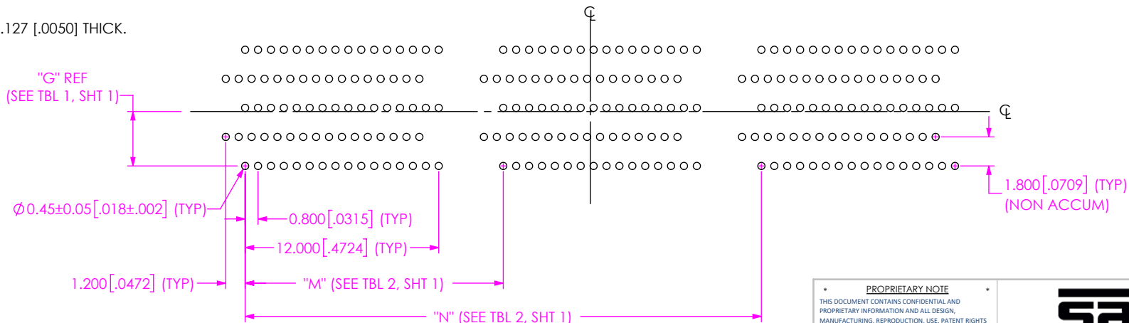
FIG 8 NVAF-DP-05-3-XX.X-X-X-K-XR STENCIL SHOWN F:\dwg\misc\mktg\footprint\NVAF-XX-XX-XX.X-X-X-K-XR-FOOTPRINT.slddrw
