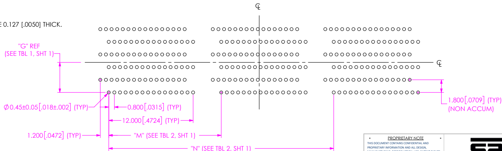
FIG 10 NVAF-DP-06-3-XX.X-X-X-K 1 XR STENCIL SHOWN F:\d\wg\misc\mktg\footprnt\NVAF-XX-XX-X-XX.X-X-X-K 1 XR-FOOTPRINT.slddrw
