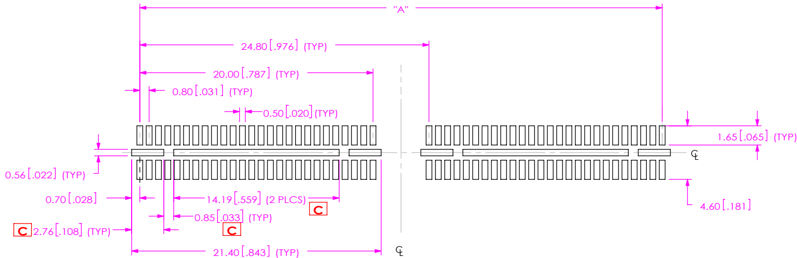
FIG 2 C QRF8-052-XX.X-X-D-A SHOWN
