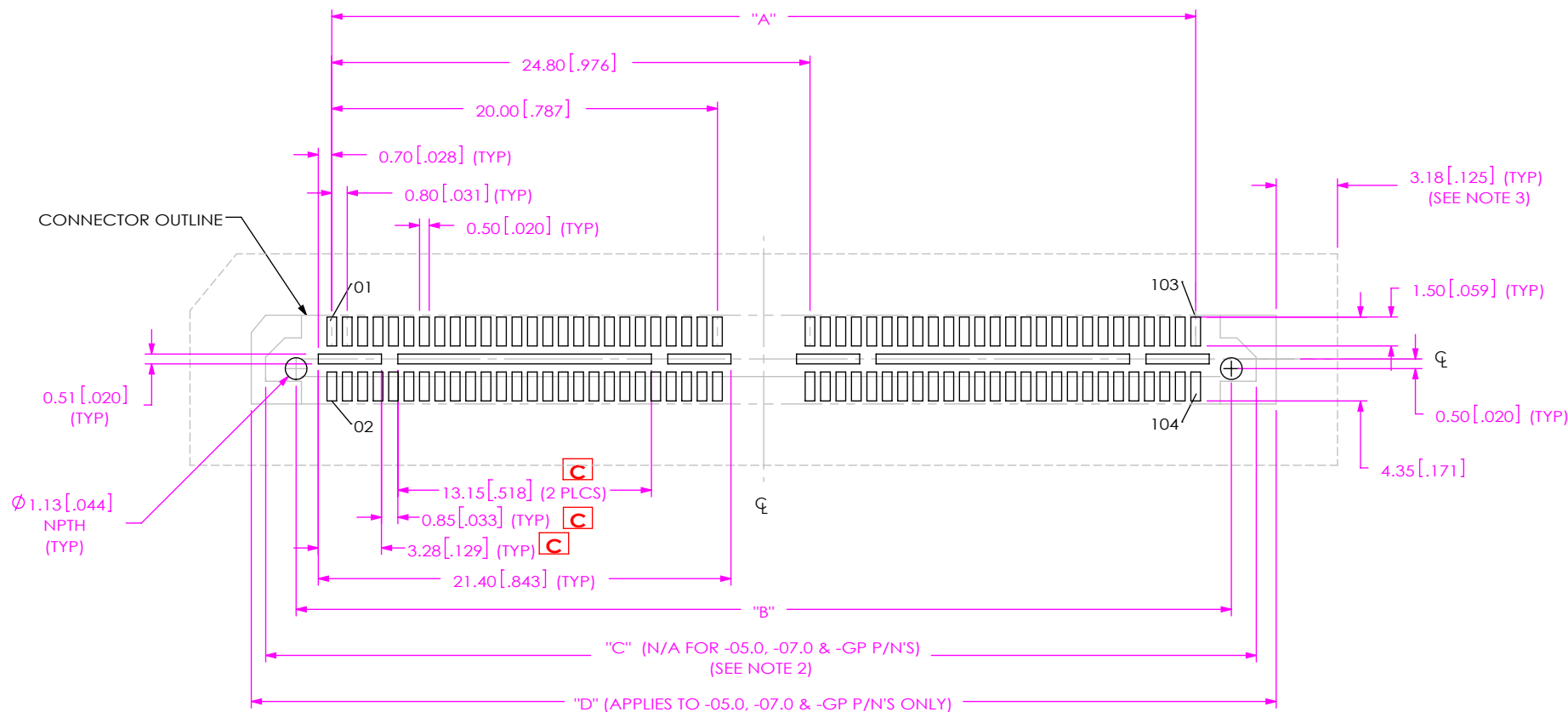
FIG 1 C QRM8-052-XX.X-X-D-A SHOWN
