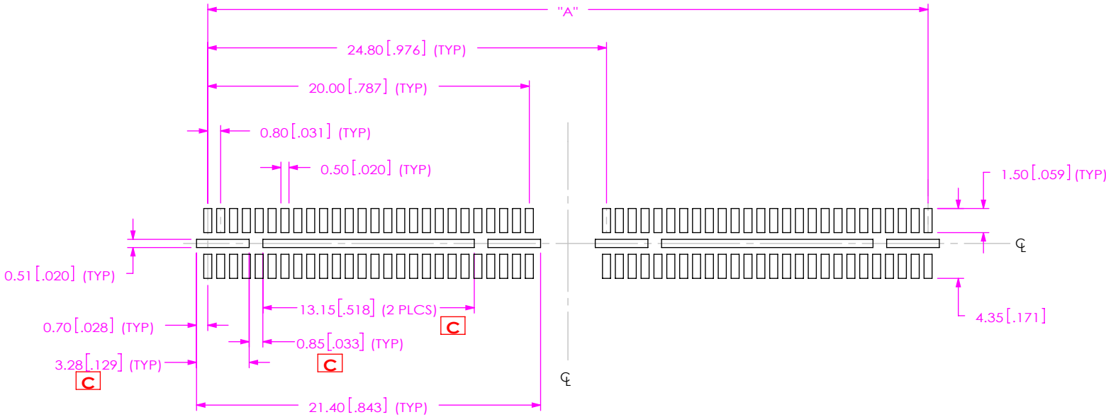
FIG 2 C QRM8-052-XX.X-X-D-A SHOWN
